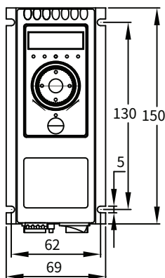
SL-30U (顶视图)
