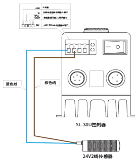
通用传感器启停控制 (NPN两线)
