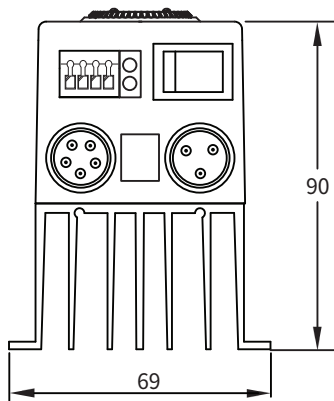
SL-30U 4.5A (正视图)
