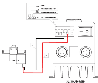
同步输出端口驱动电磁阀
