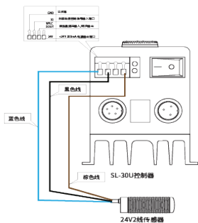
通用传感器启停控制 (NPN三线)
