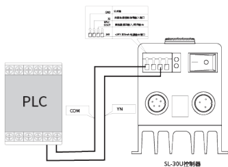
PLC模拟量输出做输出电压控制
