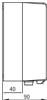
SL-30U 4.5A (左视图)
