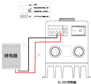
同步输出端口驱动继电器
