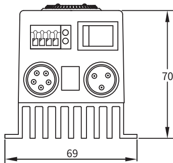
SL-30U 3A (正视图)
