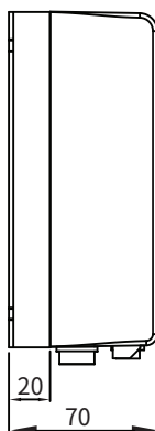
SL-30U 3A (左视图)
