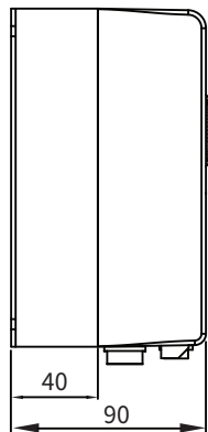
SL-30F 4.5A (左视图)
