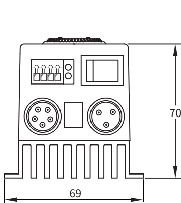
SL-30F 1.5A 3A (正视图)
