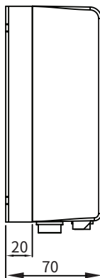
SL-30F 1.5A 3A (左视图)
